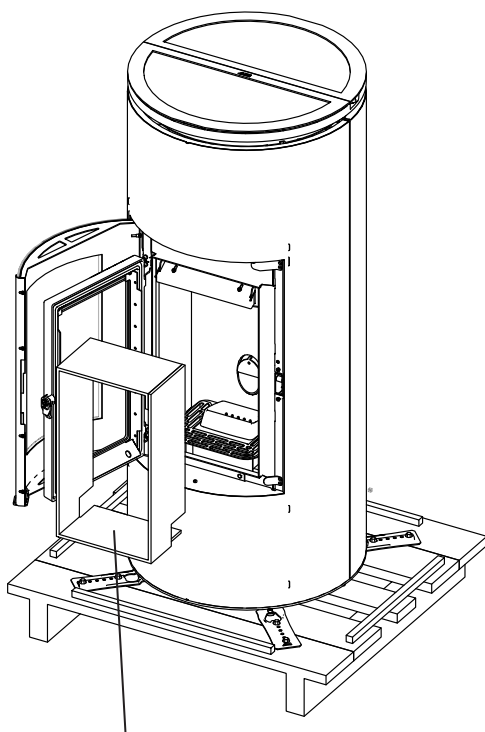
ÔTER LE CARTON CONTENANT LES PLAQUES EN FONTE DU FOYER
