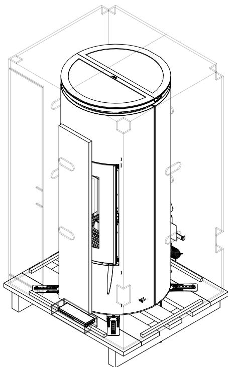
EMBALLAGE POÊLE MOOD
